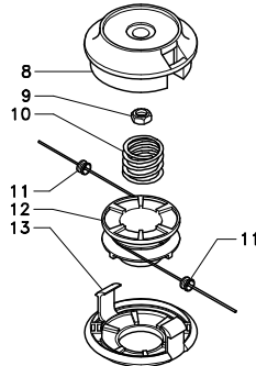
"FLASH RAPID" 14(8+13)
